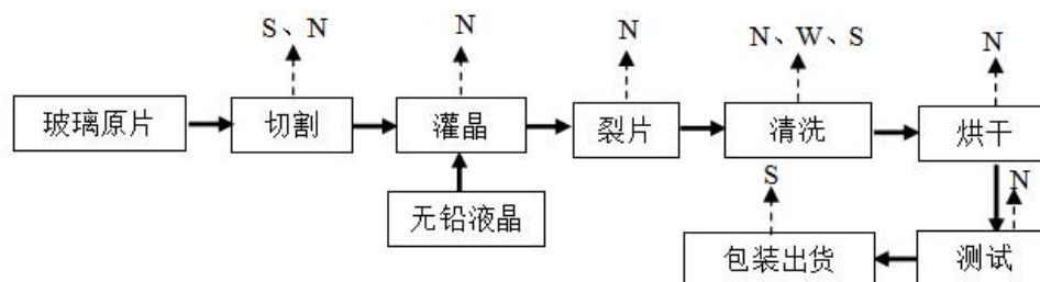
图 3-3 项目生产工艺及产污环节流程图
